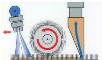
Sistema iniezione-estrazione
